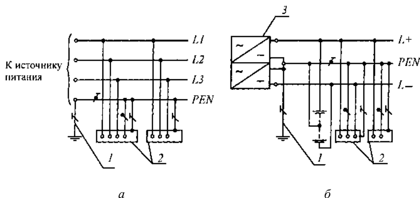
Рис. 1.7.1. Система TN-C переменного ( а ) и постоянного ( б ) тока. Нулевой защитный и нулевой рабочий проводники совмещены в одном проводнике: 1 - заземлитель нейтрали (средней точки) источника питания; 2 - открытые проводящие части; 3 - источник питания постоянного тока
