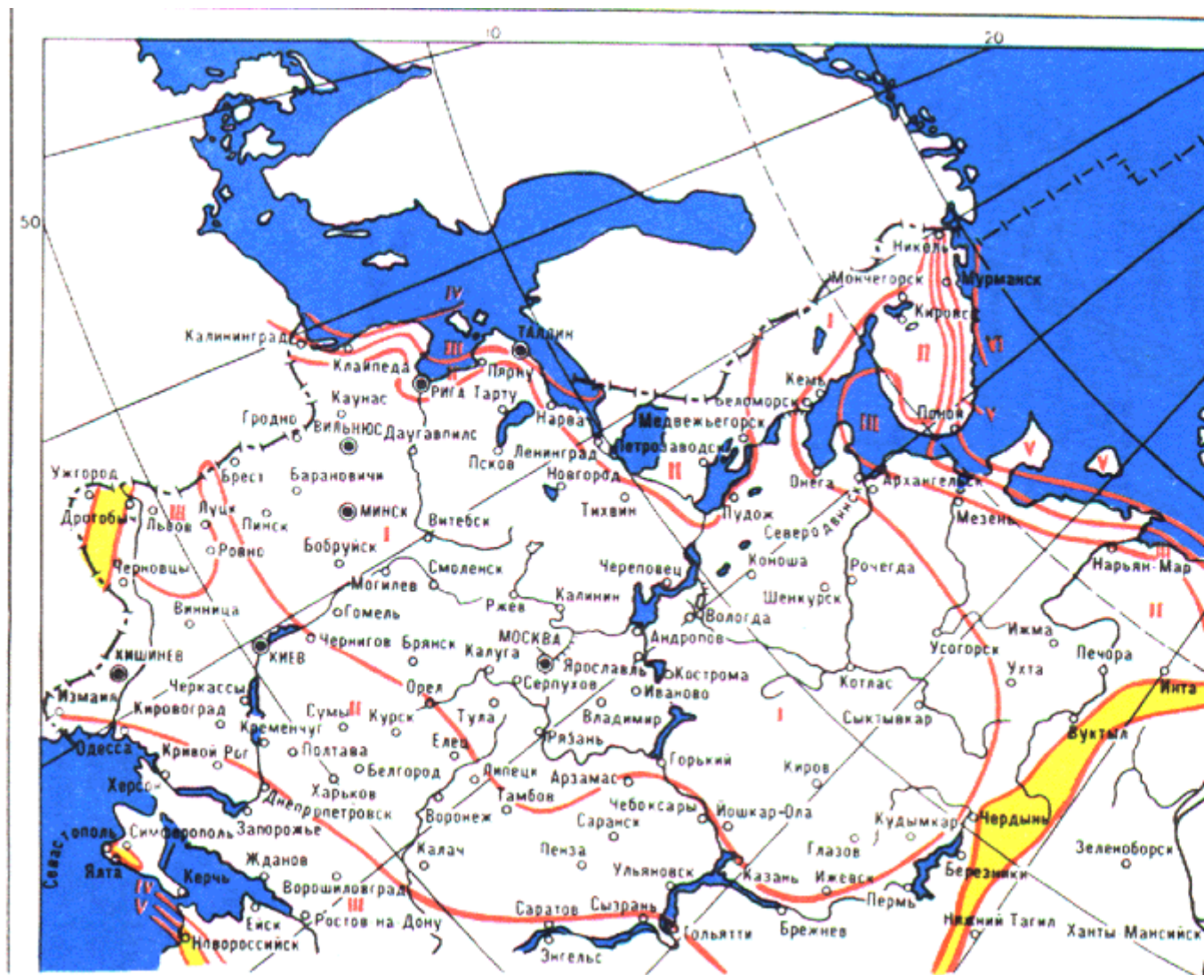
Рис. 2.5.1. Карта районирования территории СНГ по скоростным напорам ветра. Лист 1
