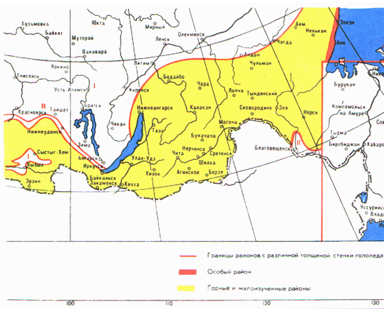
Рис. 2.5.8. Карта районирования территории СНГ по толщине стенки гололеда. Лист 4
