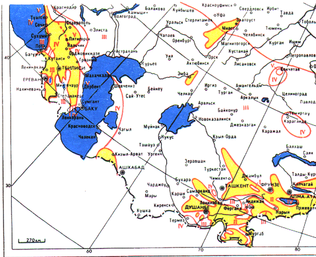
Рис. 2.5.2. Карта районирования территории СНГ по скоростным напорам ветра. Лист 2
