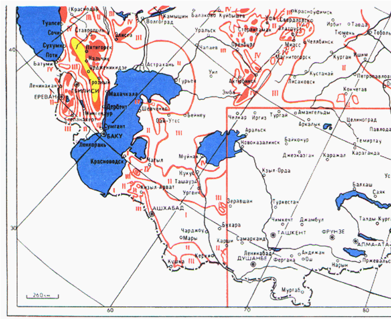
Рис. 2.5.6. Карта районирования территории СНГ по толщине стенки гололеда. Лист 2
