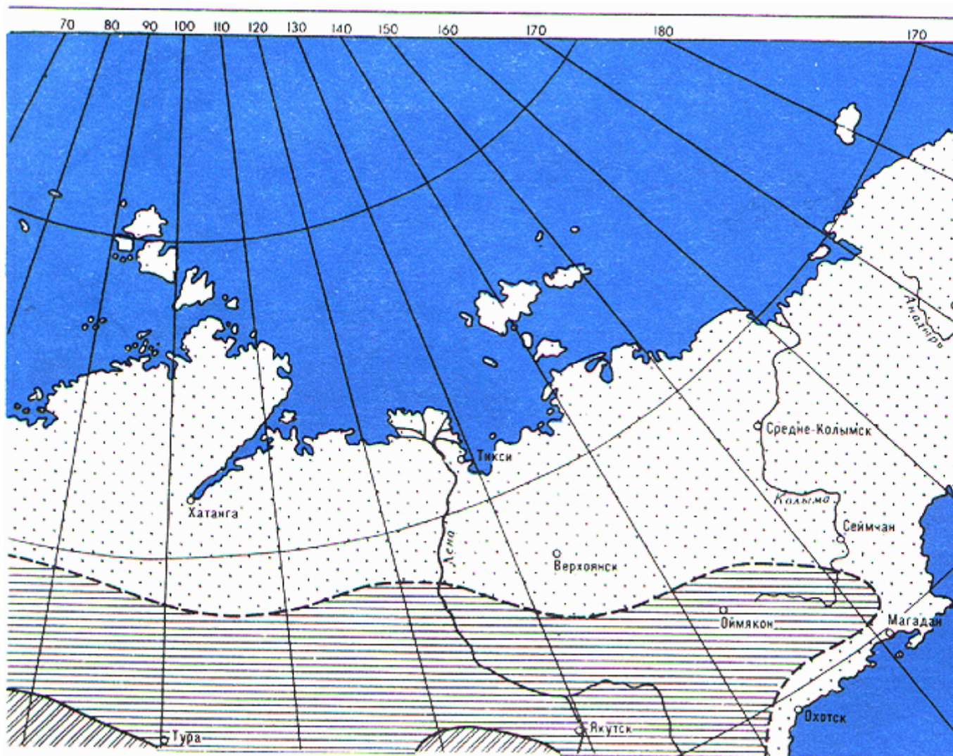
Рис. 2.5.15. Карта среднегодовой продолжительности гроз. Лист 3
