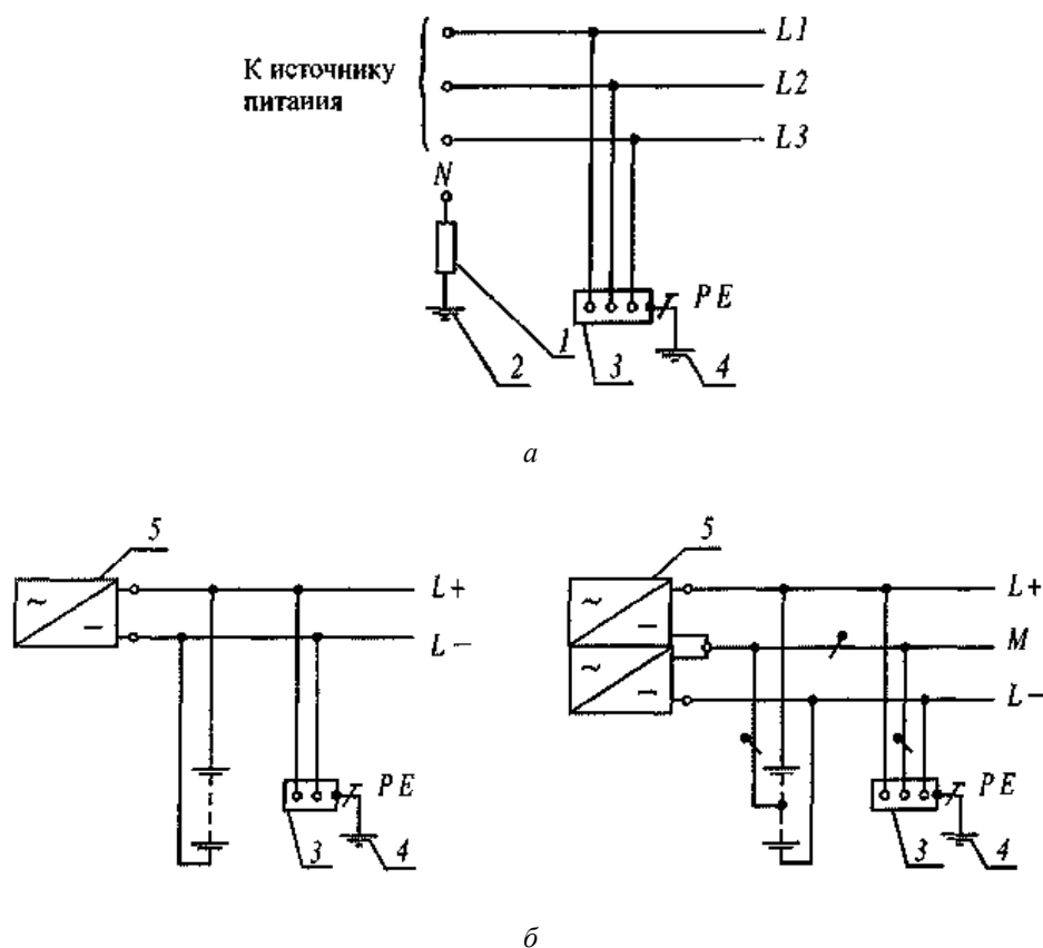
Рис. 1.7.4. Система ИТ переменного (а) и постоянного (б) тока. Открытые проводящие части электроустановки заземлены. Нейтраль источника питания изолирована от земли или заземлена через большое сопротивление:
