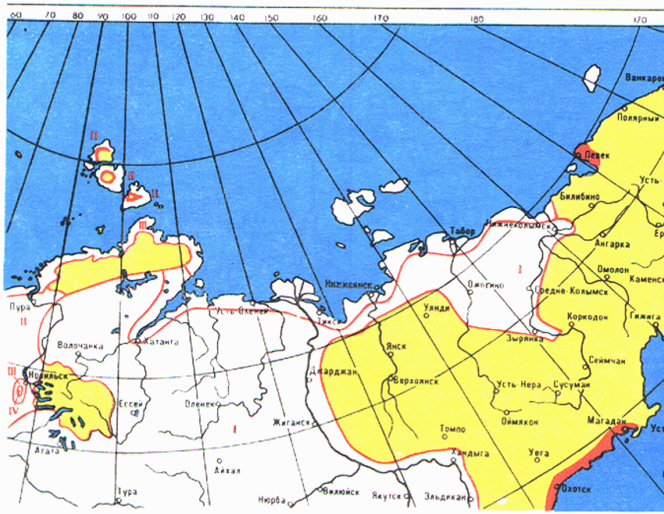
Рис. 2.5.7. Карта районирования территории СНГ по толщине стенки гололеда. Лист 3
